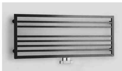
AVENTO AVFLA horizontální provedení antracit 905 × 480 mm
