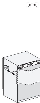
FNS7040E, FNS7040B, FNS7040C, FNS7040D, built-in (*footnote) (installation drawings)
