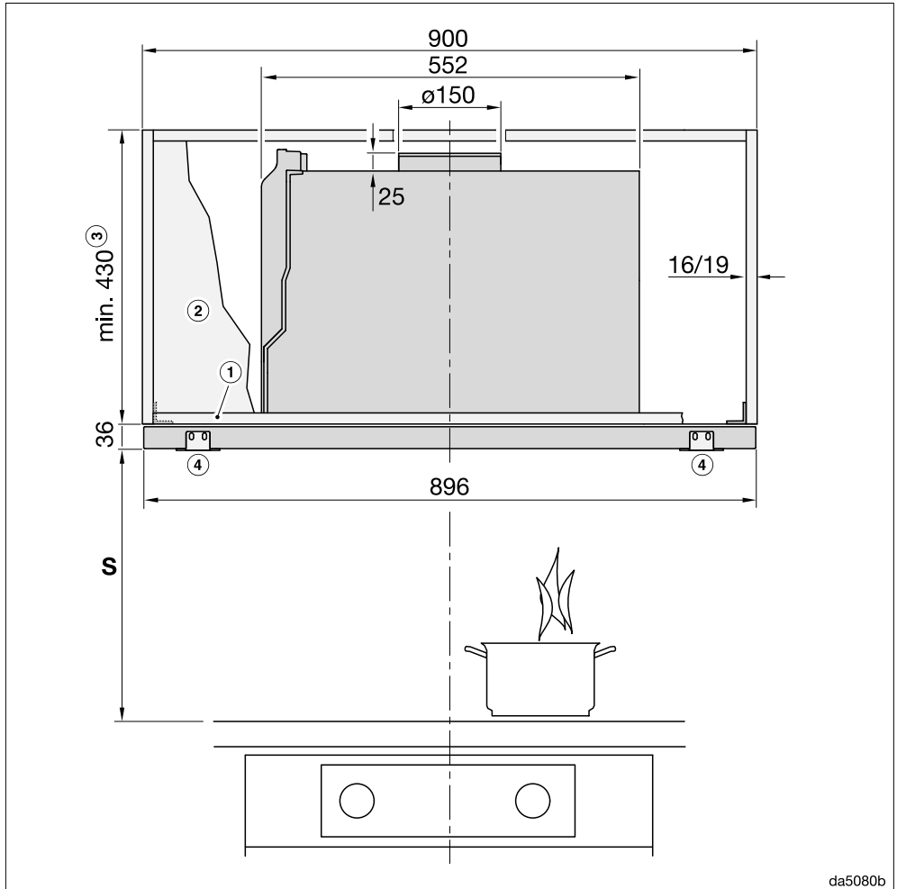
Obr. 2: DAS 4920 ve skříni široké 900 mm.
