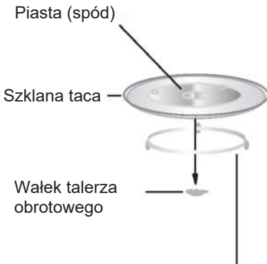
Montaż pierścienia talerza obrotowego
