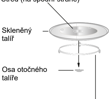
Sestava otočného prstence
