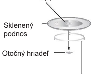
Zostava otočného krúžku
